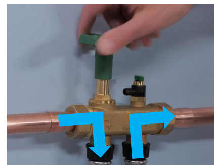
Position ouverte (Volant dévissé)
